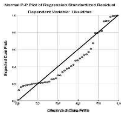
Gambar 4.2 Grafik P-Plot
