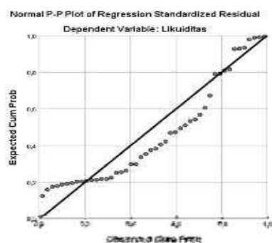
Gambar 4.2 Grafik P-Plot
