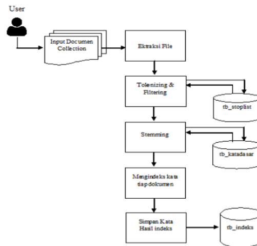
Gambar 1. Skema proses input koleksi dokumen
