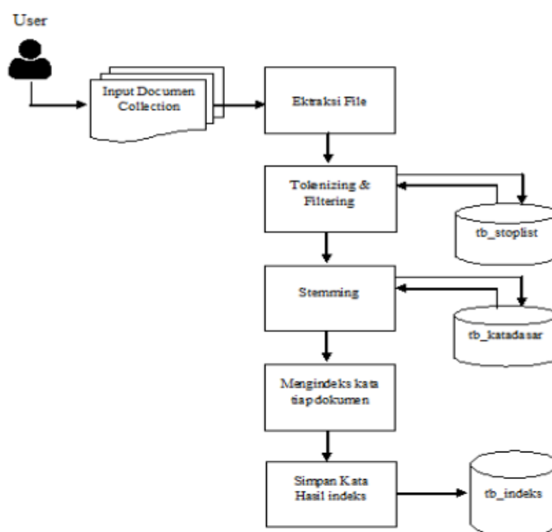
Gambar 1. Skema proses input koleksi dokumen
