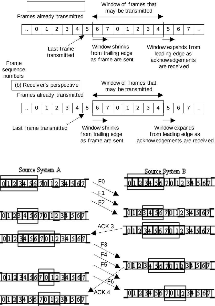
Gambar 3.9 Mekanisme sliding windows beserta contoh transimisi message
