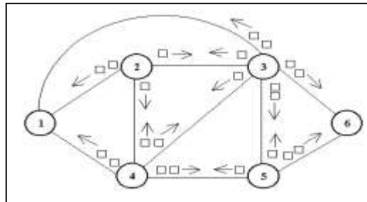
Gambar 4.11. Hop ketiga
