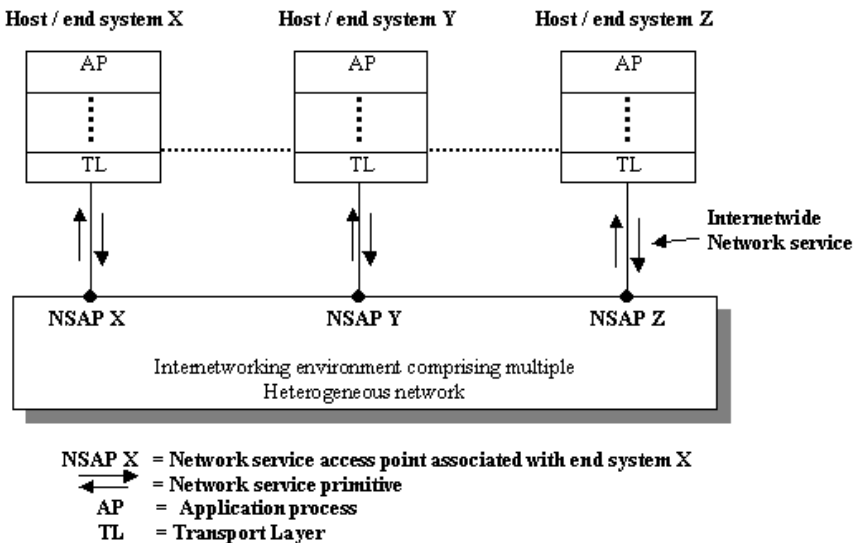
Gambar 4.17 Skema pelayanan jaringan internet
