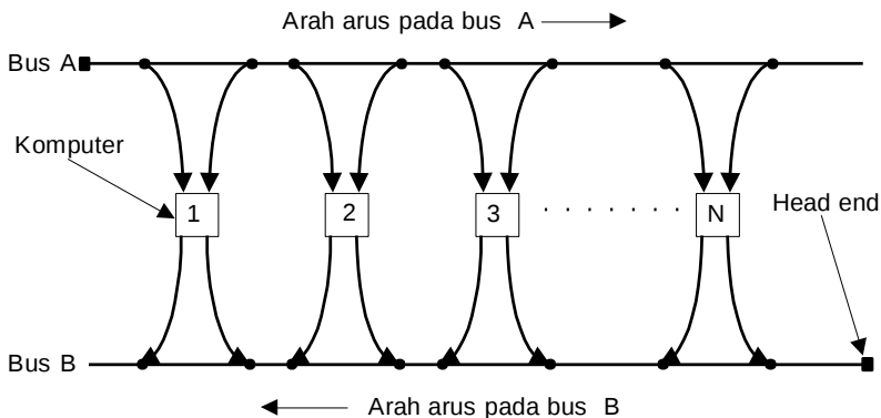
Gambar 1.3 Arsitektur MAN DQDB
