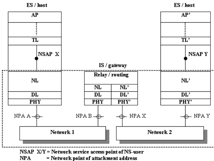
Gambar 4.18 Hubungan antara alamat NSAP dan NPA
