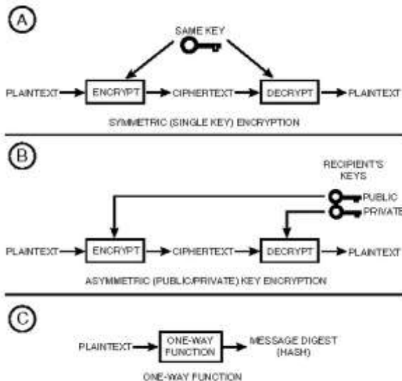
Gambar 5.3 Tiga teknik kriptografi
