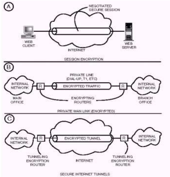
Gambar 5.4. Tiga tipe kanal aman yang dapat memberikan kerahasiaan data.
