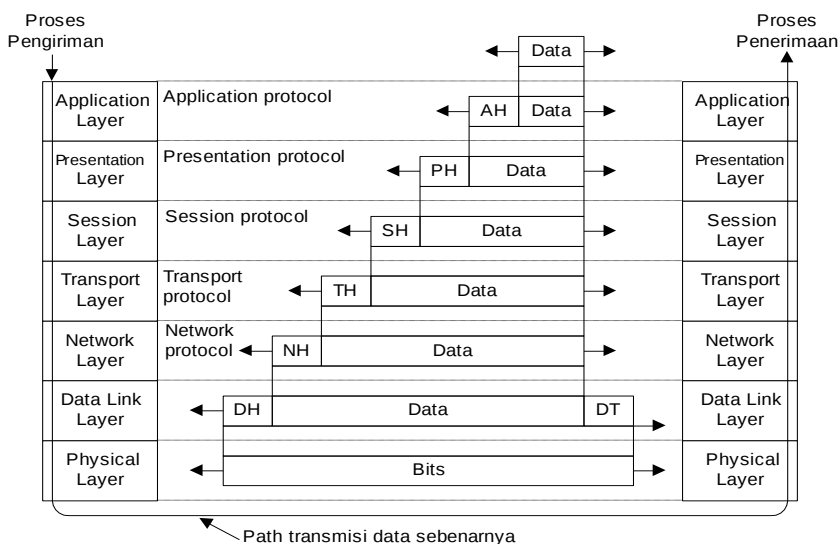
Gambar 2.2 Contoh tentang bagaimana model OSI digunakan
