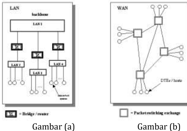
Gambar 4.15. Arsitektur internetwork
