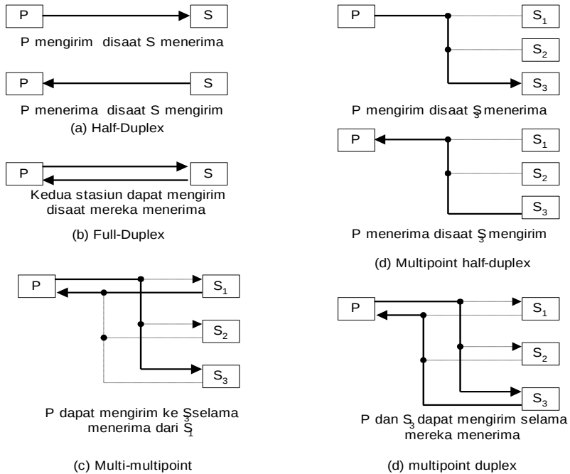
Gambar 3.2 Hubungan konfigurasi saluran
