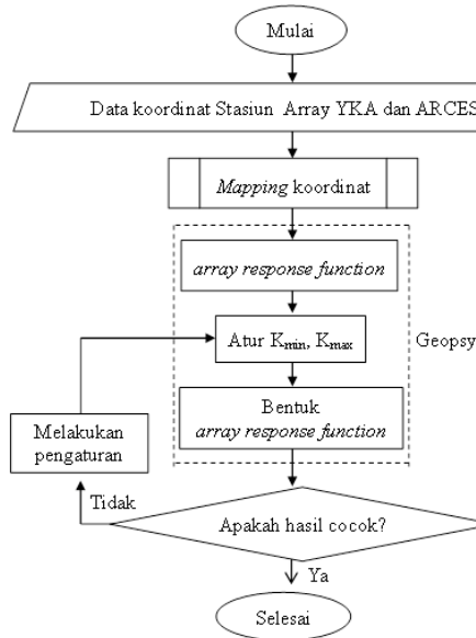
Gambar 3. Diagram alir proses pengujian bentuk array response function
