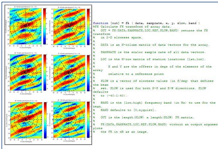
Gambar 7. Pergerakan energy maksimum dalam array response function setiap 10 detik selama 40 detik yang menunjukkan pergerakan rekahan disertai listing program matlab.
