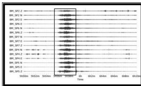
Gambar 5. Hasil rekaman seismogram utuh keseluruhan data rekaman,
