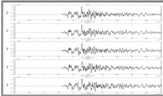
Gambar 6. Data Rekaman yang telah mengalami proses filter dan restitusi, sehingga menjadi semakin jelas dimana letak event gempanya.
