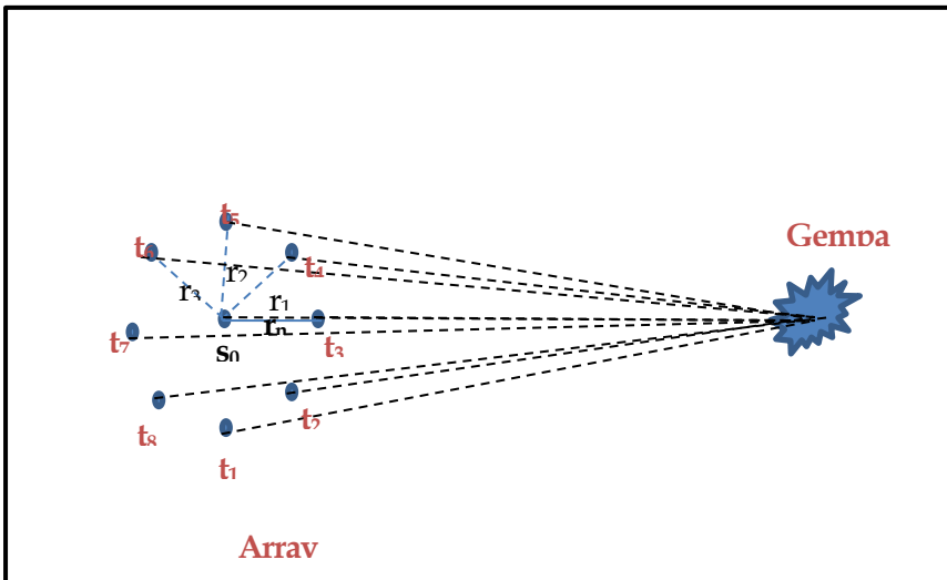
Gambar 2. Ilustrasi sinyal gempa diterima array dengan waktu tiba yang berbeda beda yaitu t_1, t_2, t_3, t_4, t_5, t_6, t_7 dan t_8 tergantung dengan jarak yang terdekat dan terjauh dengan episentrum gempa, r_n adalah jarak dari pusat array dengan stasiun array lainnya dan s_0 merupakan slowness pada pusat array.
