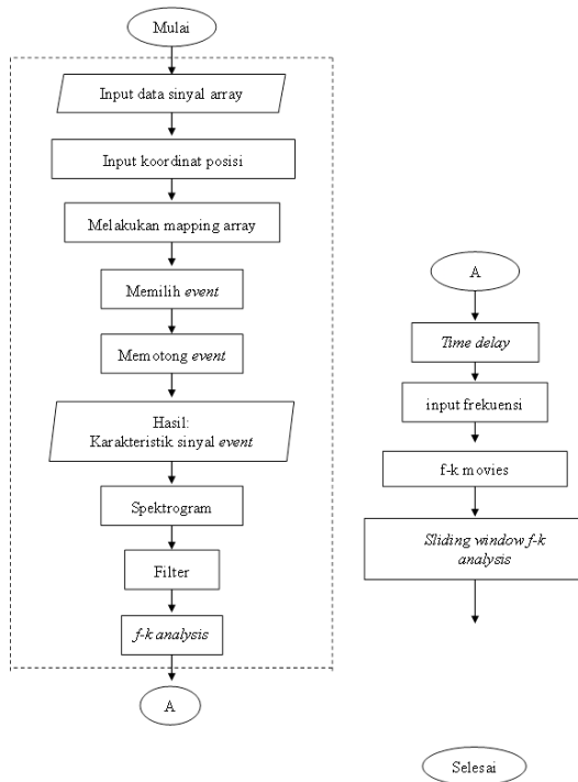
Gambar 4. Diagram alir Pemrosesan data sinyal array.
