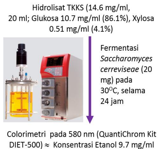
Gambar 2. Fermentasi Anaerobik dan Analisis Konsentrasi Alkohol
